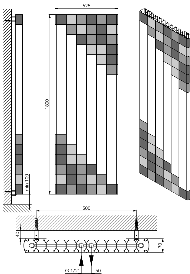
BITHERM Defile 625/1800
