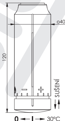
Detail regulátoru RC
