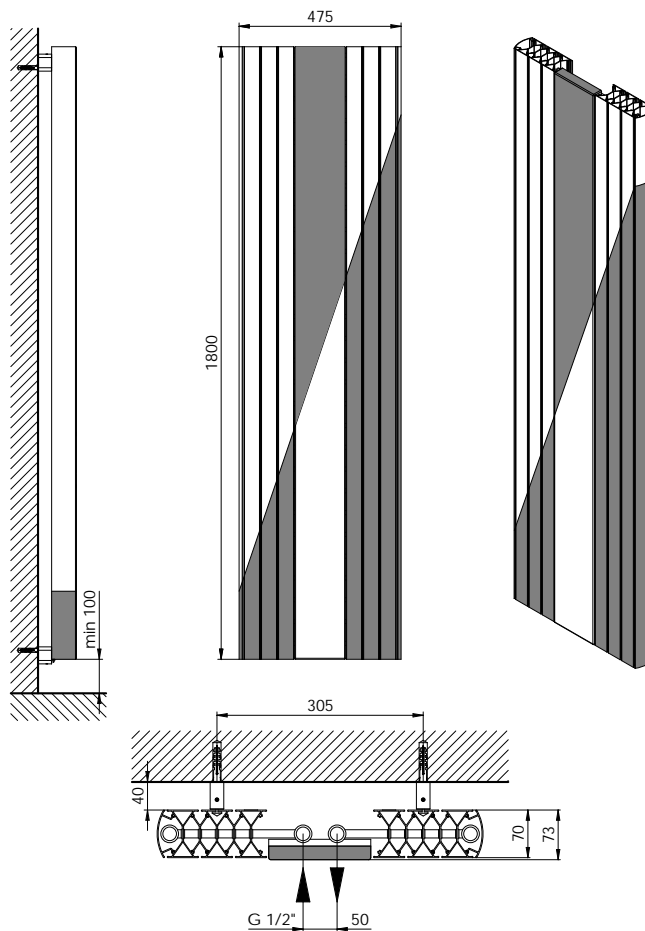
BITHERM Pierot 475/1800
